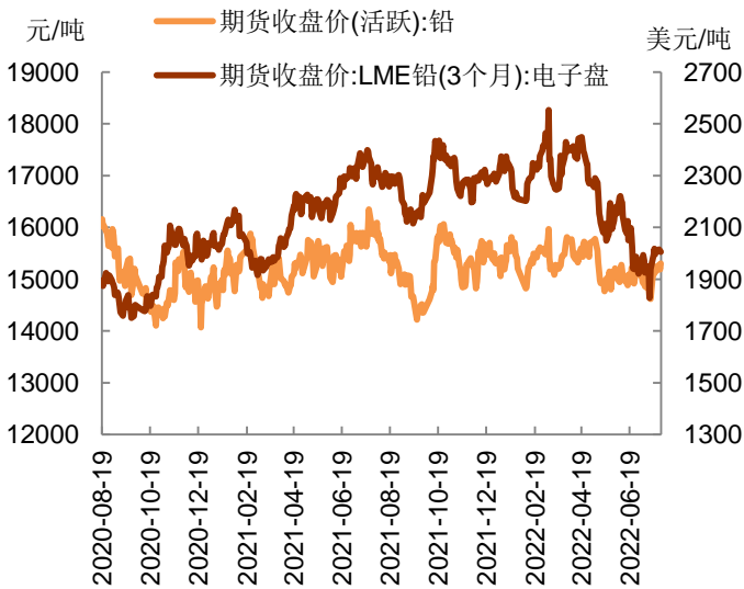
图表 1 SHFE 与 LME 铅价
