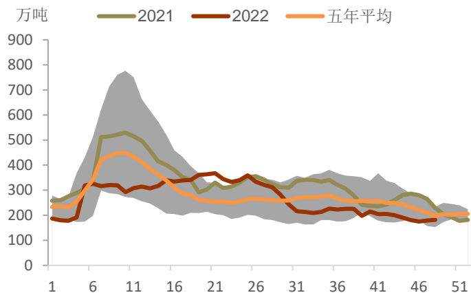
图表 13 螺纹钢厂库
