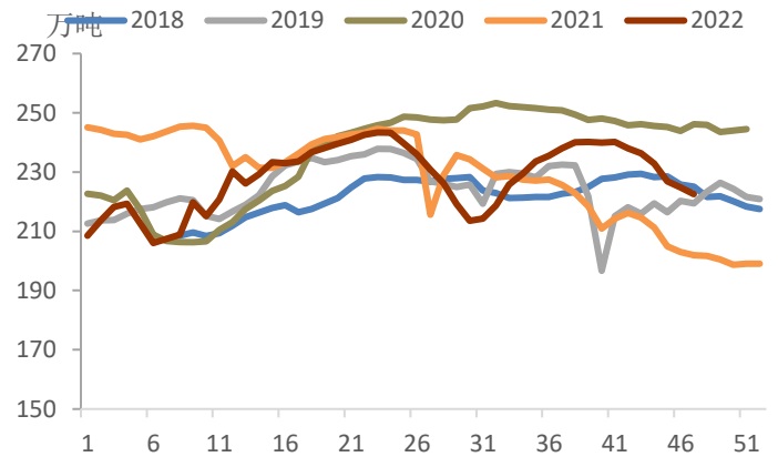
图表 20 247 家钢厂日均铁水产量
