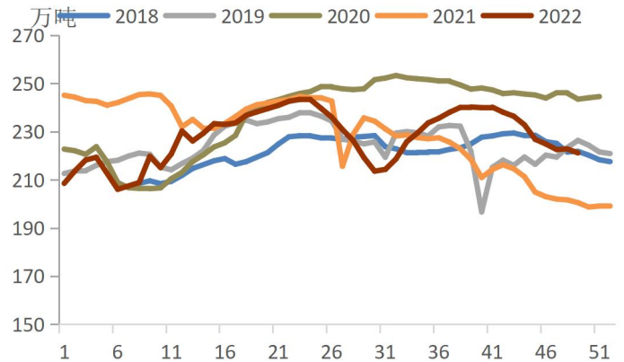
图表 20 247 家钢厂日均铁水产量
