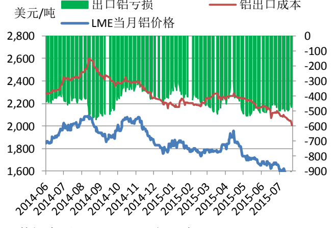
铝出口套利走势
