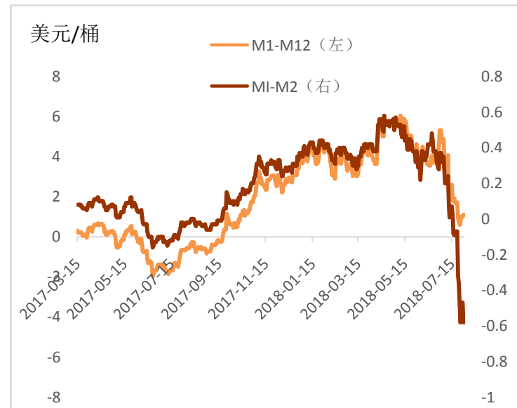
图 4 Brent 原油期货合约间价差
